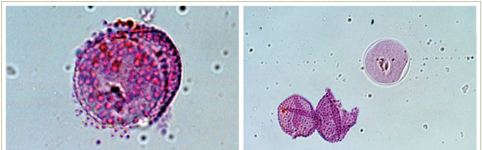
Χαρακτηριστικά γυρεόκοκκου Σχήμα: ωοειδές • Διάμετρος P: 44.8μm (37.9-47.5) • Διάμετρος E: 47.7μm (43.0-49.6)
